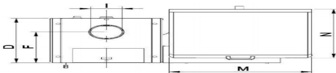
Rysunek 7.2 Wymiary kotła SMART EKO, SMART PLUS
