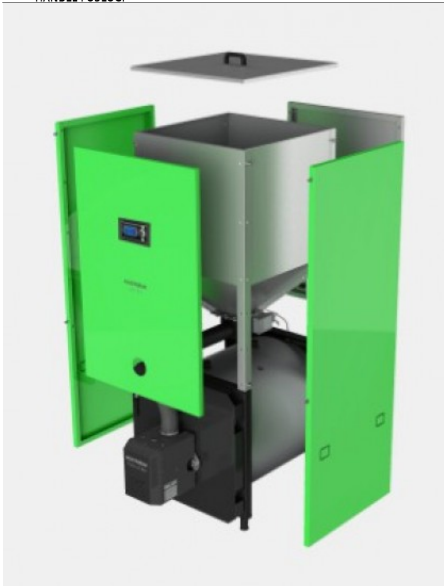
Regulator kotła Platinum Bio Ecomax 860P SIMPLE
